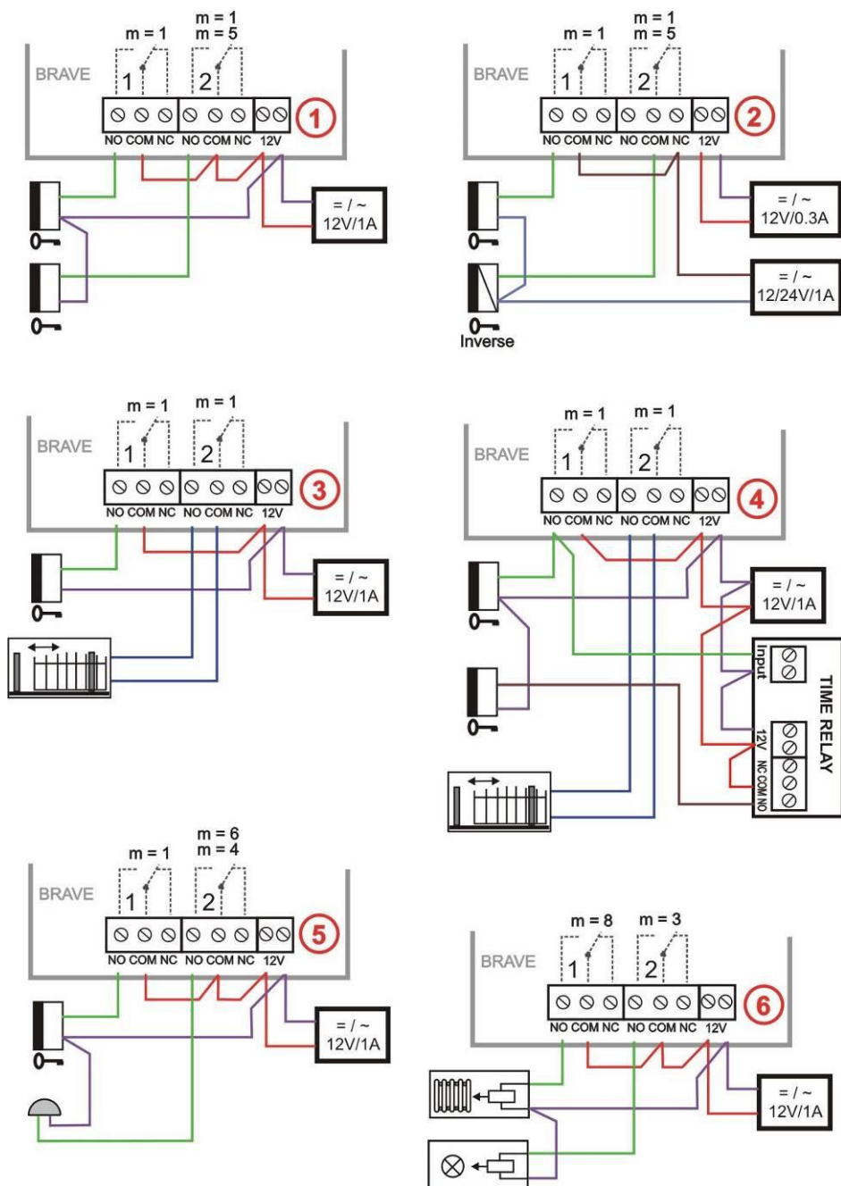
Obr. 2 Příklady zapojení spínačů
