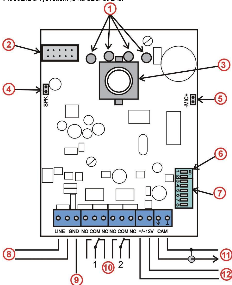
Obr. 1 Základní deska vrátného Brave Smyle
